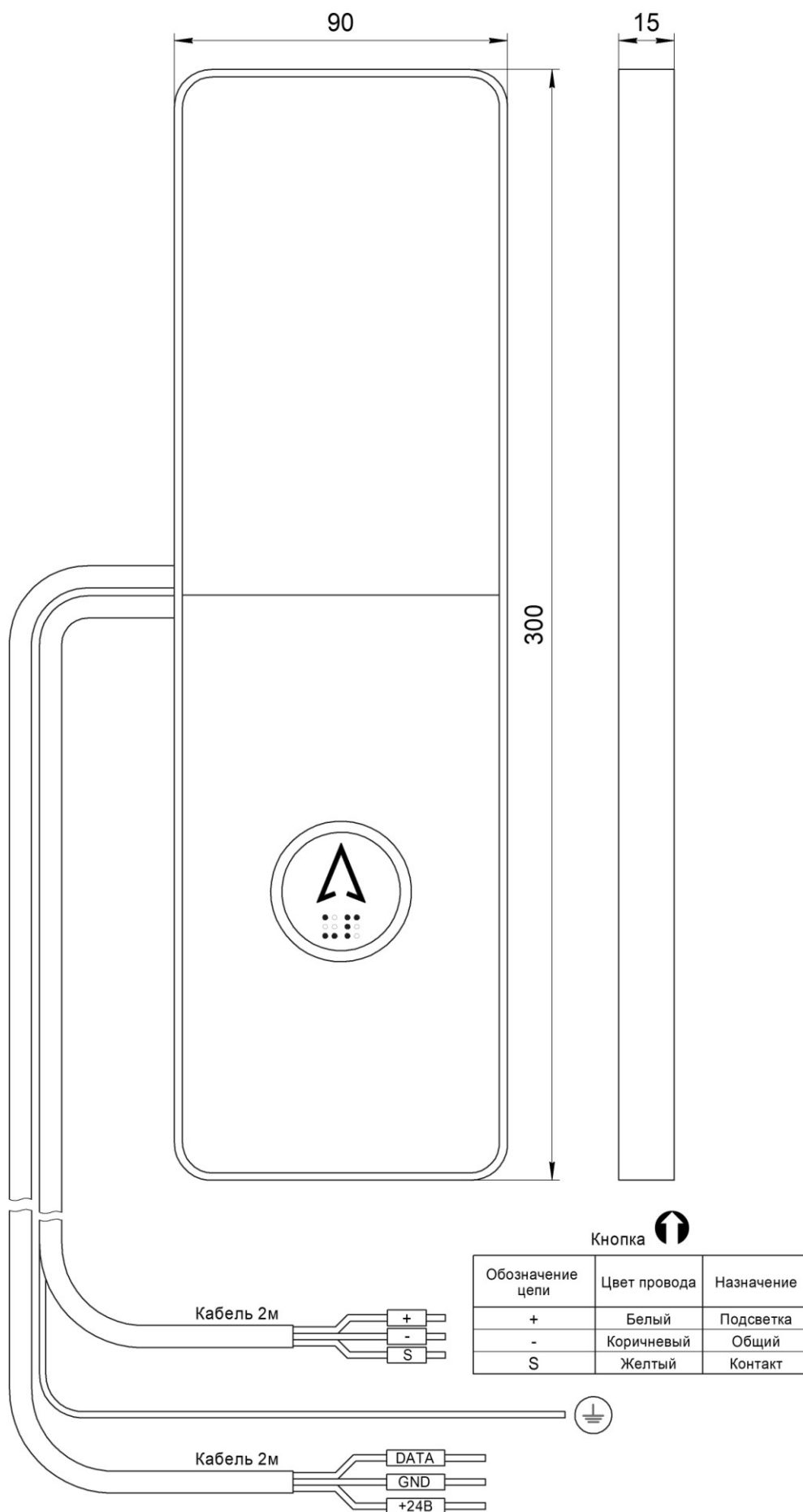
Рис.1 Внешний вид Вызывной пост GOLD (2404) НШЕК.468381.204
